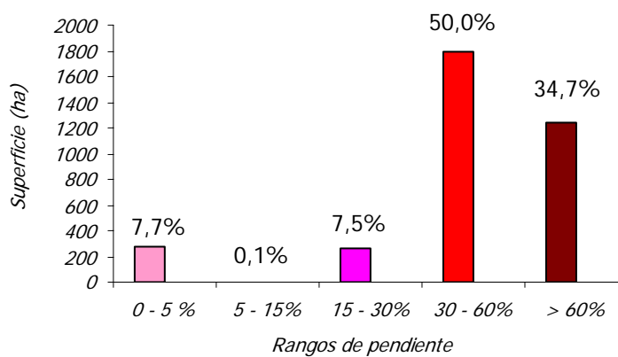
GRÁFICO 3 Distribución de la superficie del Monumento Natural del Teide según rangos de pendiente
