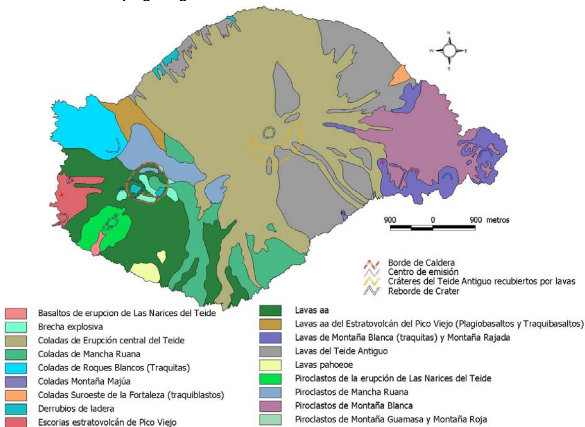
FIGURA 2 Mapa geológico del Monumento Natural del Teide.
