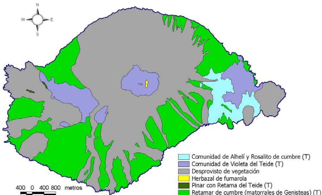
FIGURA 9 Distribución territorial de las diferentes comunidades de vegetación en el Monumento Natural del Teide
