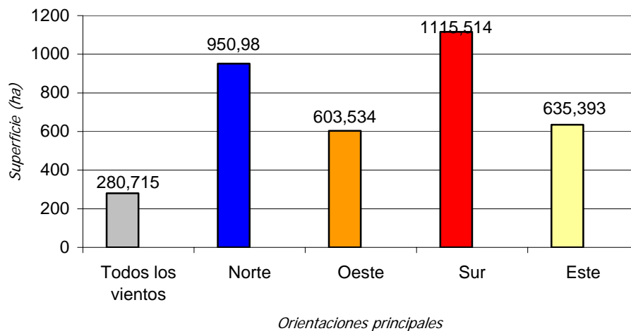
GRÁFICO 4 Distribución en superficie de las diferentes orientaciones principales del Monumento Natural del Teide
