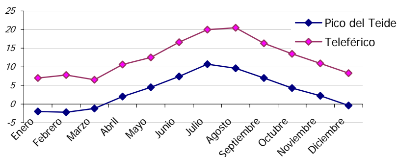
GRÁFICO 1 Evolución anual de temperaturas medias en las estaciones de Pico del Teide y Teleférico
