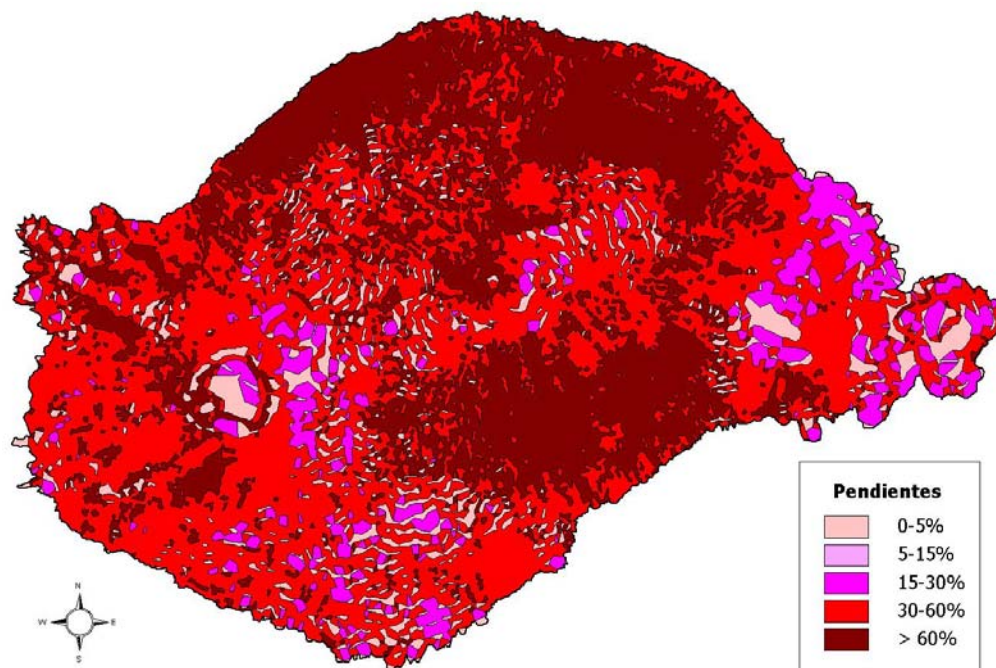
FIGURA 4 Pendientes del Monumento Natural del Teide. Vista desde el extremo suroccidental.
