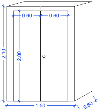
DETALLE ARMARIO ALZADO EXTERIOR
