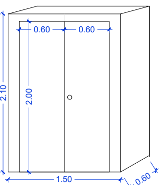
DETALLE ARMARIO ALZADO EXTERIOR
