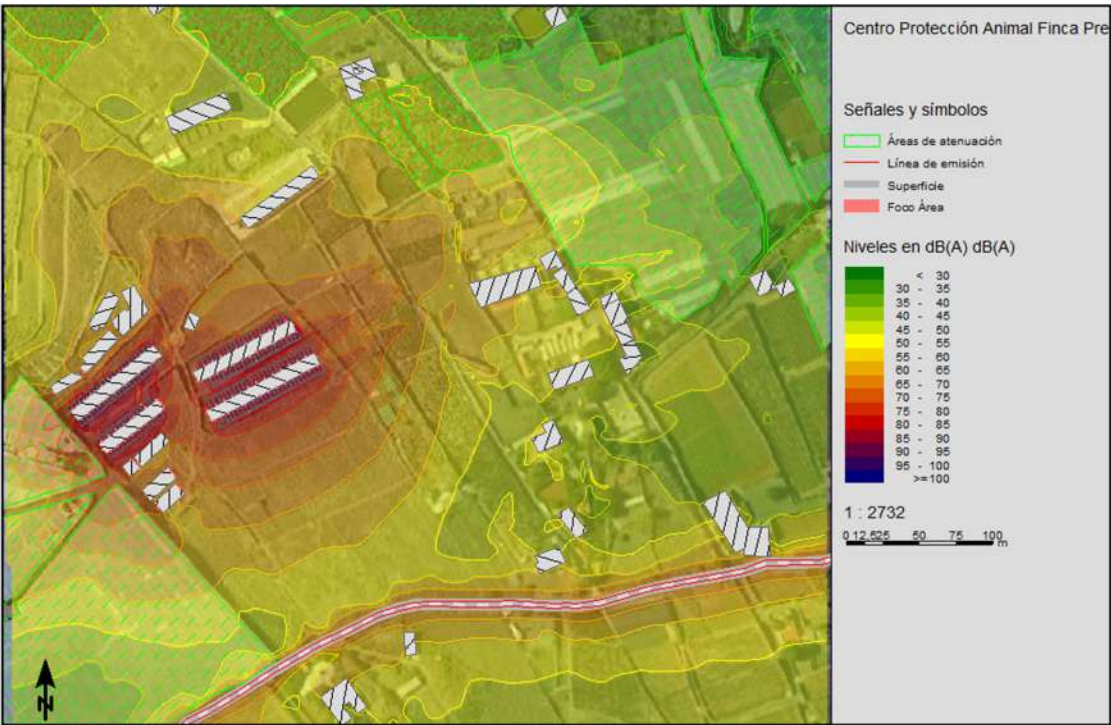
Fig 29: Propagación del ruido producido por el Centro de protección animal en periodo noche sin aplicar medidas correctivas.
