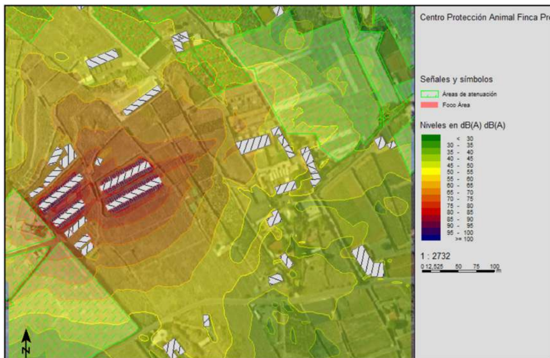
Fig 37: Mapa acústico de los niveles de ruido del "Caso 1."
