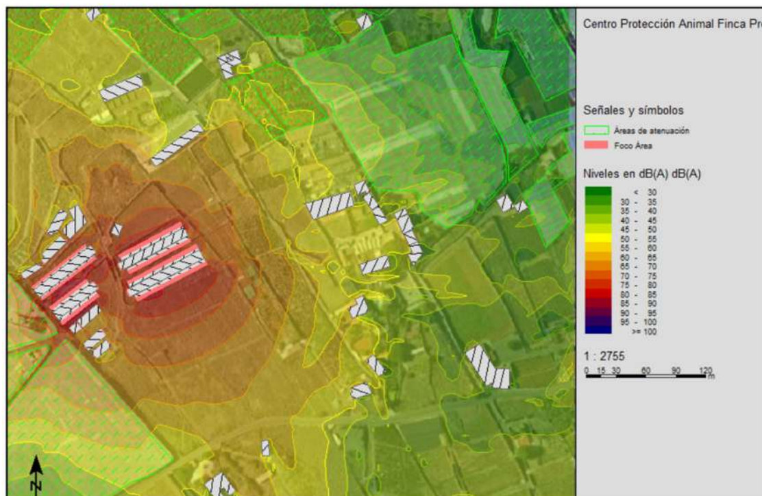
Fig 35: Propagación del ruido producido por el albergue de perros tras la modificación de su diseño original y tras aplicar las medidas correctivas.
