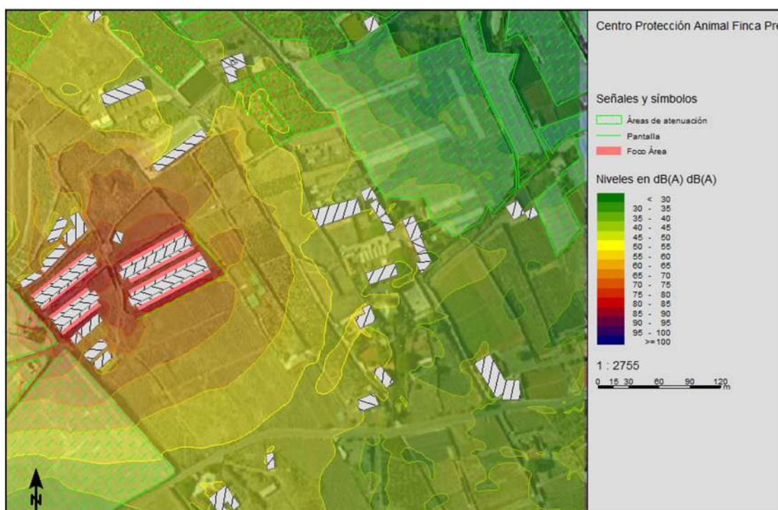
Fig 34: Propagación del ruido producido por el albergue de perros tras la modificación de su diseño original y tras aplicar las medidas correctivas.
