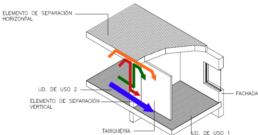
Fig 7: Esquema de vías de transmisión acústica a ruido aéreo entre dos recintos. En azul se indica la transmisión directa, a través del elemento de separación vertical. En otros colores se han indicado las transmisiones indirectas o de flancos.
