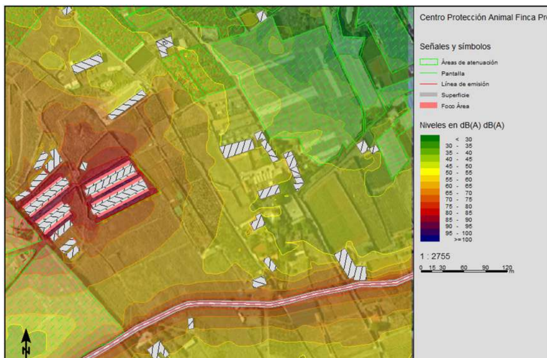
Fig 30: Propagación del ruido producido por el Centro de protección animal en periodo día tras la aplicación de las medidas correctivas.
