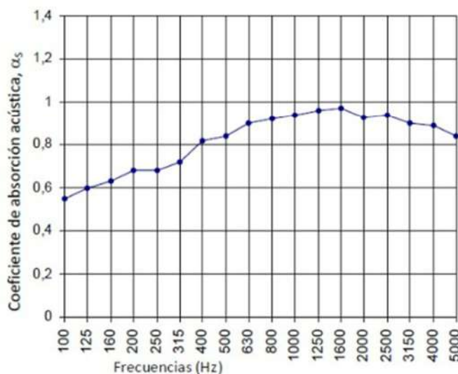
Fig 23: Ficha técnica del sistema de techo mediante panel acústico.
