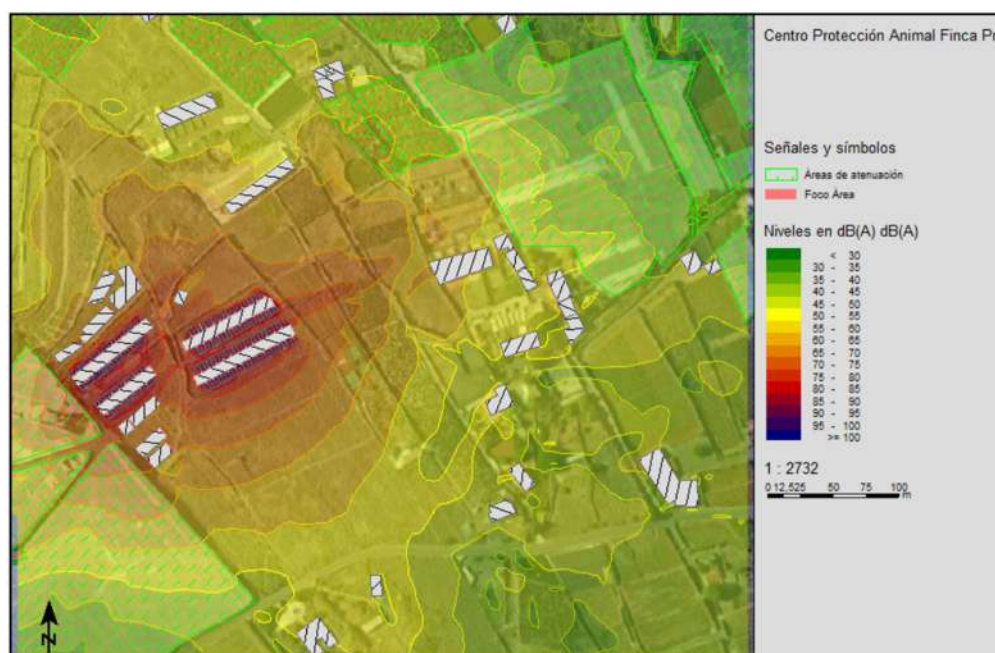
Fig 33: Propagación del ruido producido por el albergue de perros con su diseño original sin aplicar medidas correctivas.
