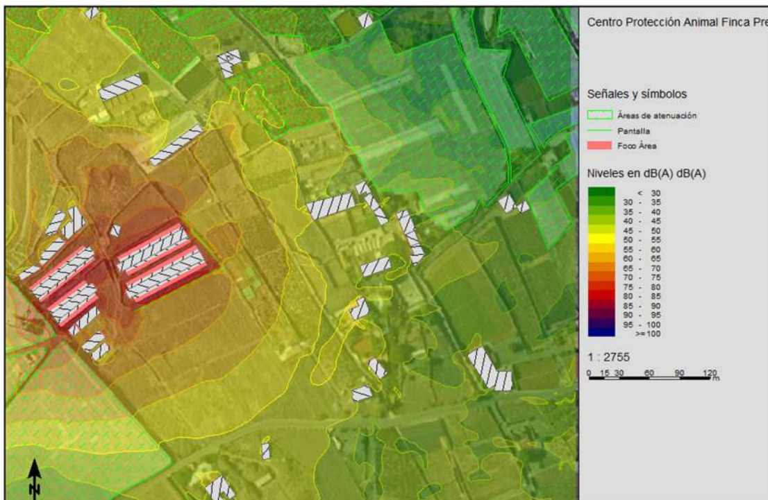
Fig 38: Mapa acústico de los niveles de ruido del "Caso 2."
