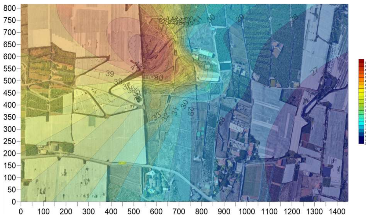
Fig 18: Mapa de ruido de los niveles de ruido actuales en periodo noche.
