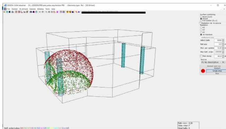
Fig 6: Vista 3D de un modelo predictivo interior.
