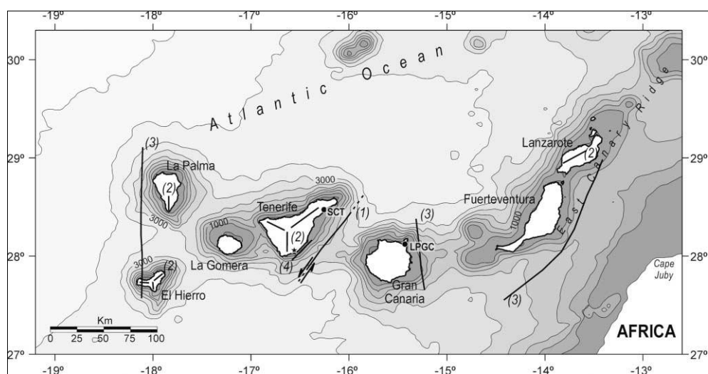
Principales estructuras y lineamientos volcánico – tectónicos del Archipiélago Canario. González Vallejo et al. (2006) 2
