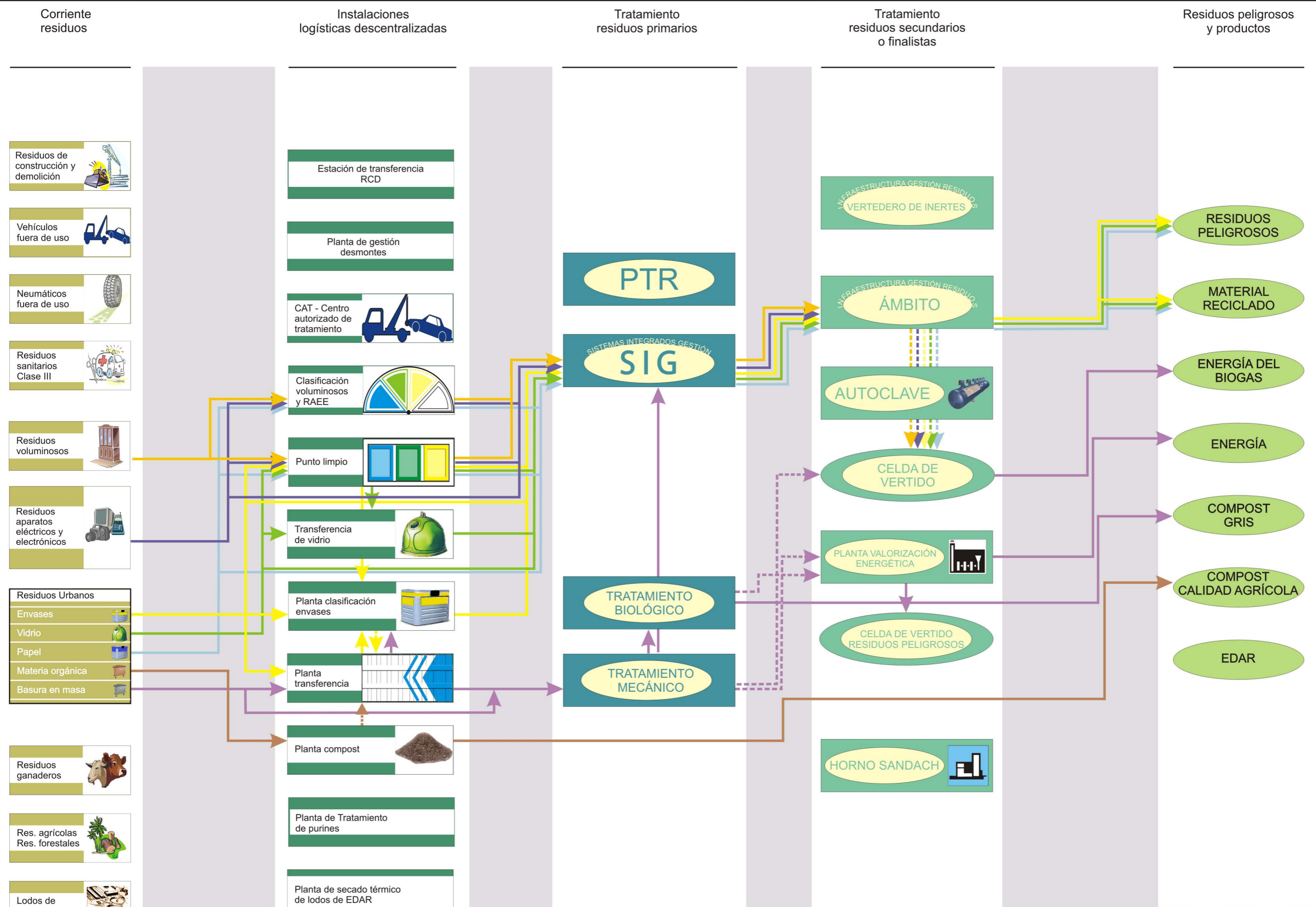
ESQUEMA DE FLUJOS DE LAS CORRIENTES DE RESIDUOS Flujo de los Residuos Urbanos RU(-)
